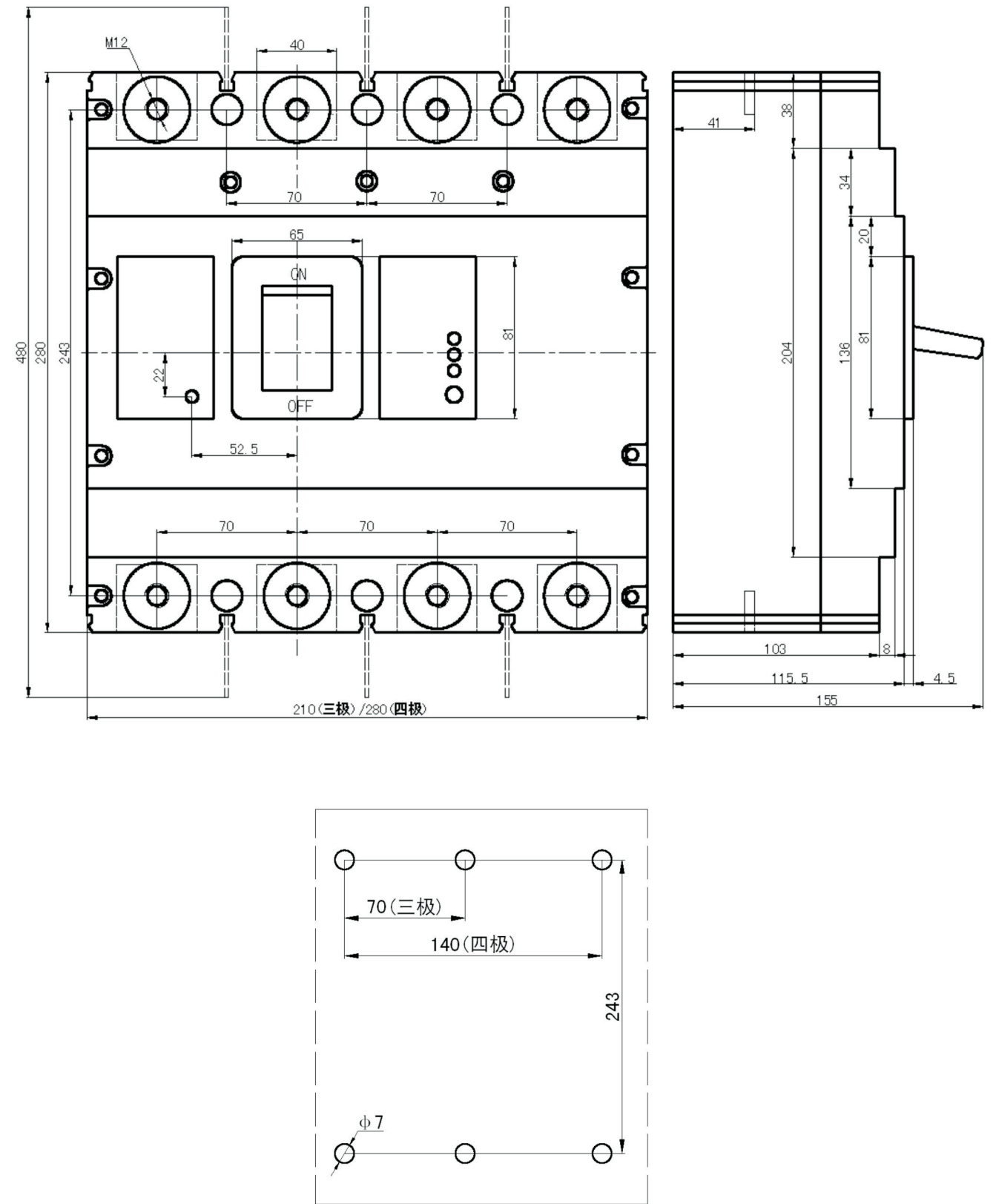
CKM33L-630板前接线
