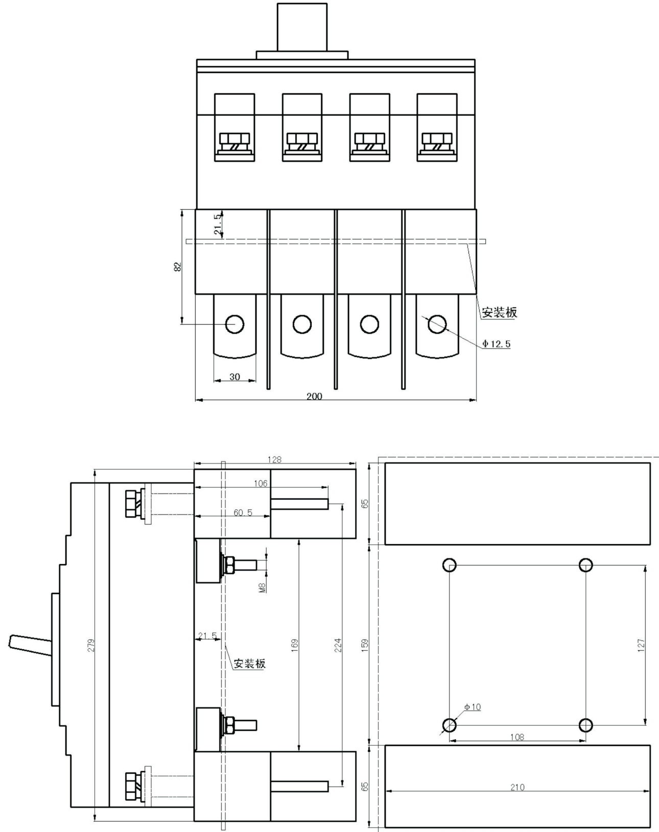
CKM33L-400插入式板后接线
