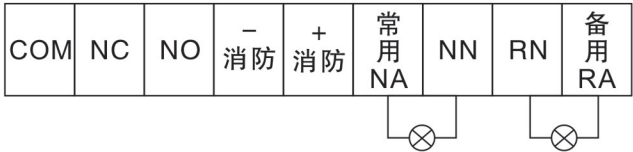
附图三 一体式3极、4极转换开关接线端
