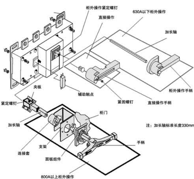
图1 安装示意图
