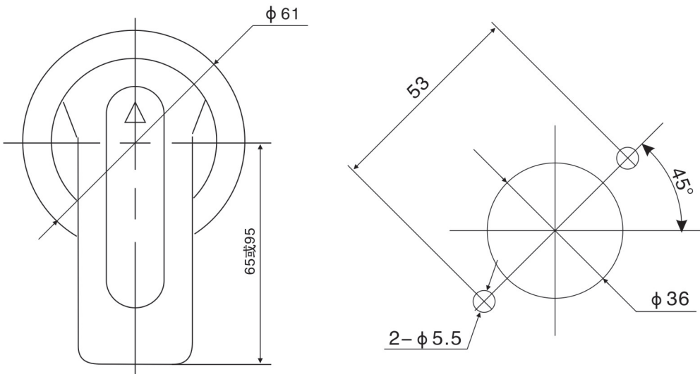
“A”型圆形手柄外形及门板开孔尺寸
