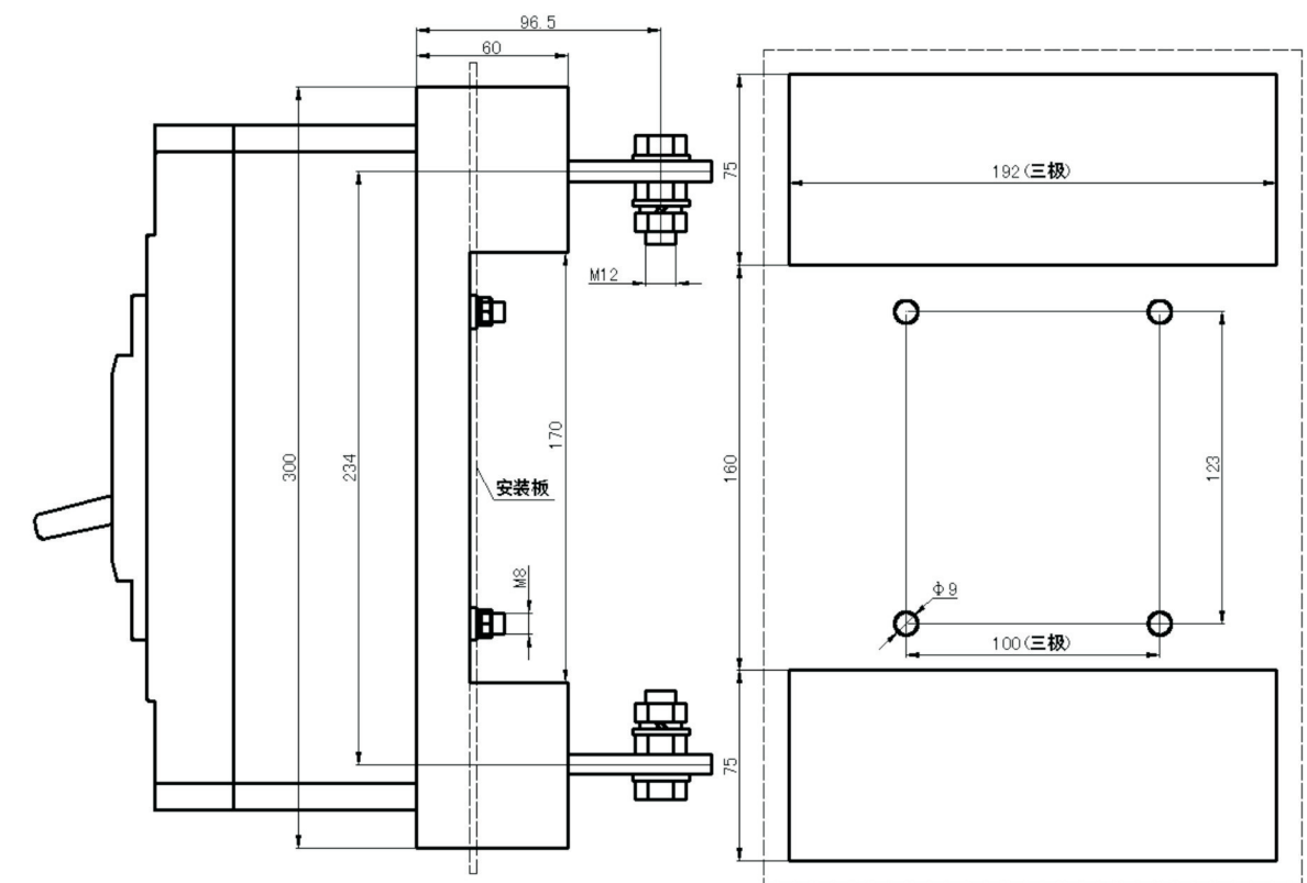
CKM55-630C、L、M插入式板后接线(3极)
