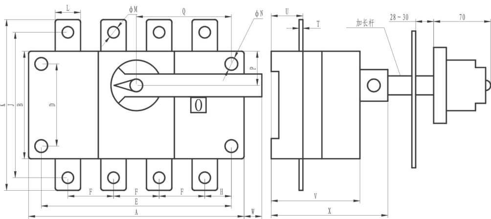
CKG33-160~630柜外操作
