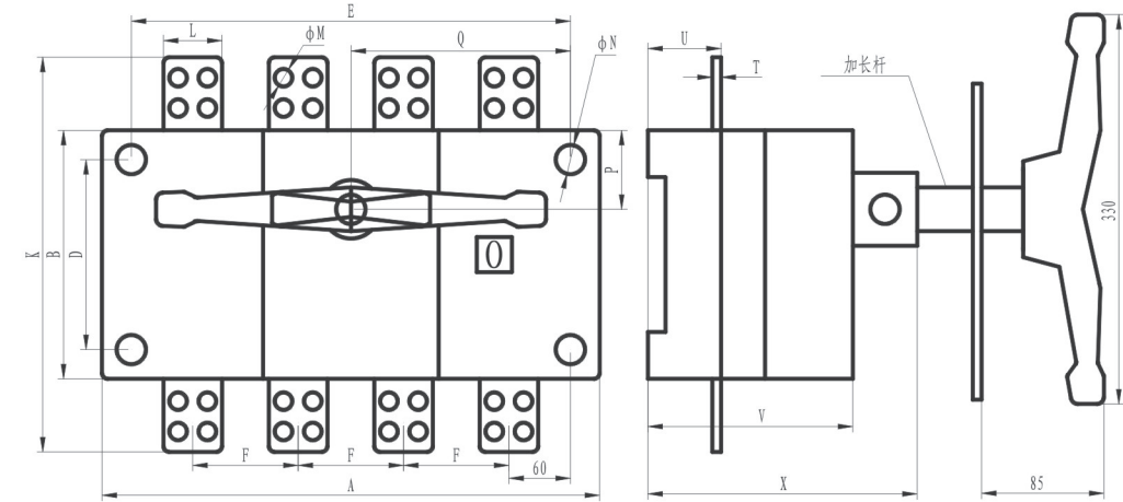
CKG33-1600柜外操作
