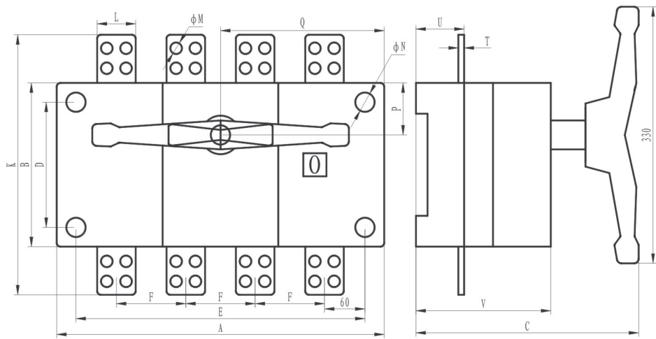
CKG33-1600柜内直接操作
